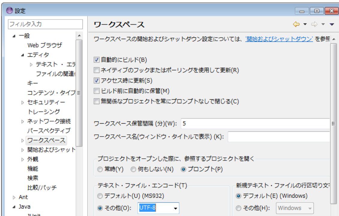
図 2.10 ソースファイルのデフォルトコードの設定
