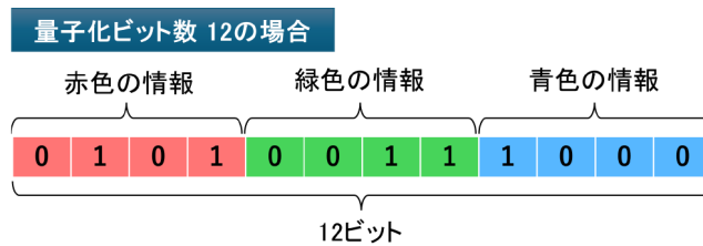
図 4.12 動画データの仕組み
